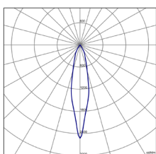
RXC-130-16°-26W
