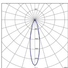
RXC-130-24°-26W
