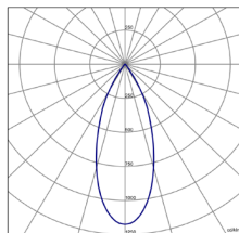
RXC-130-38°-26W
